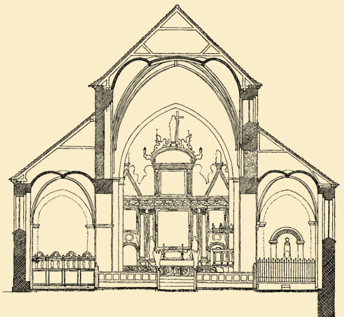
Fig. 13 Tværsnit af kirken set mod øst. Bemærk hovedskibets lave murkrone i forhold til overhvælvingen. I syd ses en stor niveauforskel mellem kirkegulv og klostergård. Her er lavet en stor terrænregulering. Opmåling: Charles Christensen 1925.
