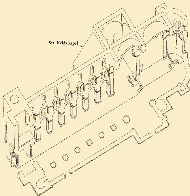
Fig. 14 Isometrisk rekonstruktion af Viborg Domkirke efter den første færdiggørelse o. 1225-50. Rekonstruktion: Jens Vellev 1982.
